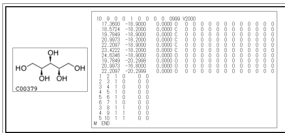
図 3.1: KEGG COMPOUND で取得できる構造式と MOL ファイルの例
