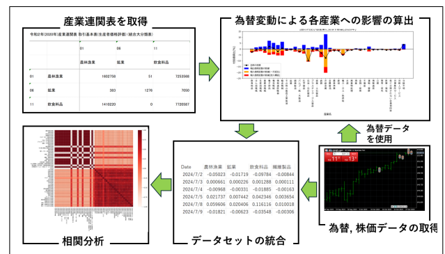
図 4.6: 相関分析の流れ
