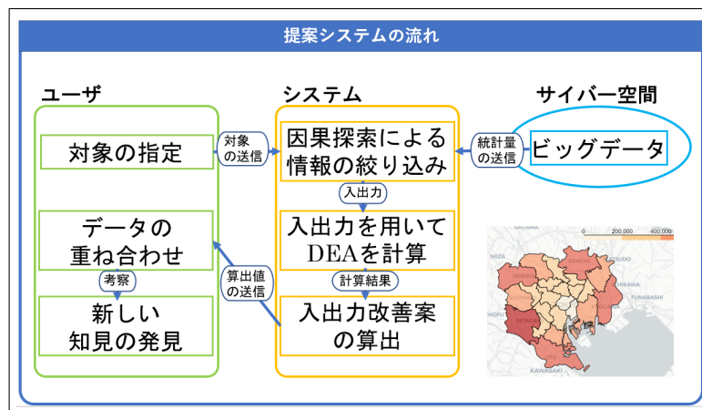
図 4.4: DEA 部分におけるシステムのフロー
