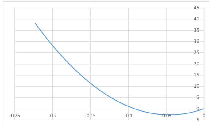
図 4 目標在庫とリードタイム
