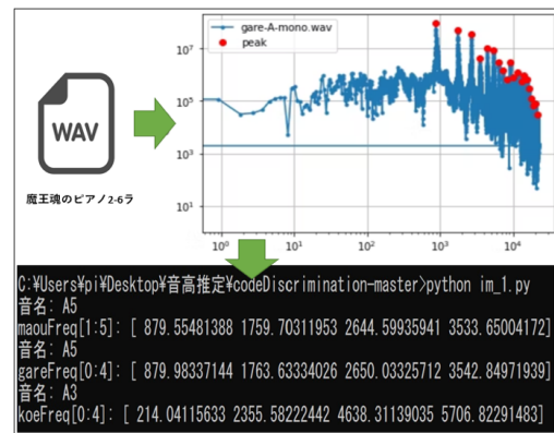
図 2.8: FFT による音高推定
