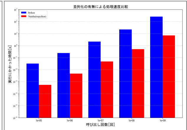
図 4.4: 並列化の有無の比較
