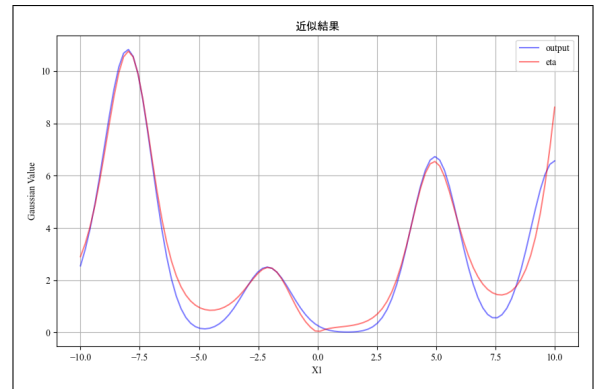
図 5.8: 学習終了時の近似結果
