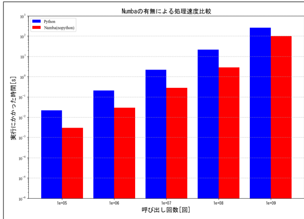
図 4.3: Numba の有無の比較
