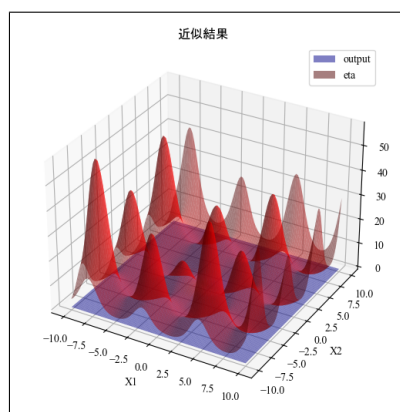
図 5.11: 1 回目の近似結果
