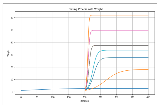
図 4.2: 複製された基底関数の重みの変化
