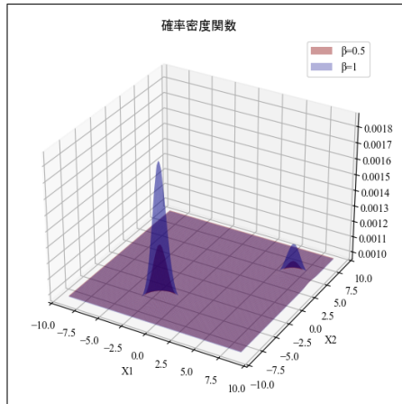
図 2.5: \mathbf{m} の条件付き確率密度関数
