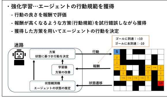
図 3.1: 強化学習の仕組み
