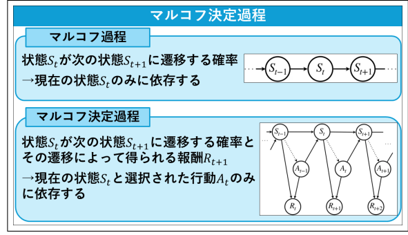
図 3.2: マルコフ過程とマルコフ決定過程
