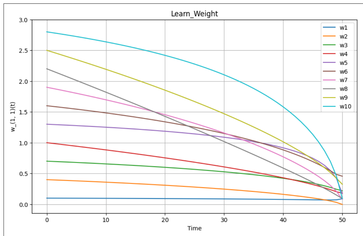
図 2.5: 数值実験
