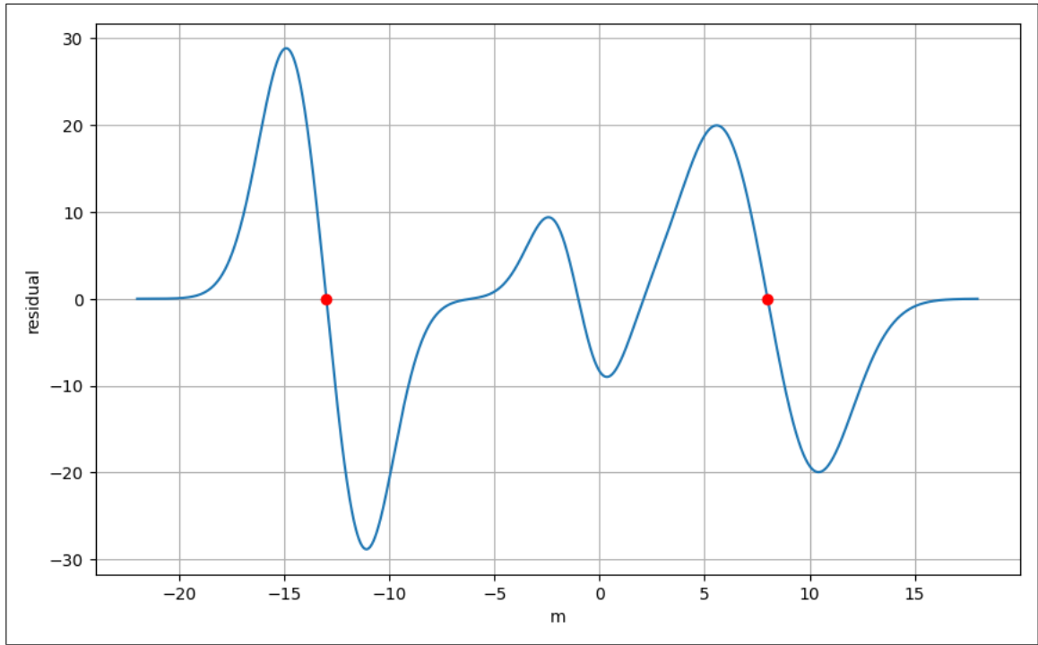
図 2.1: 数値実験
