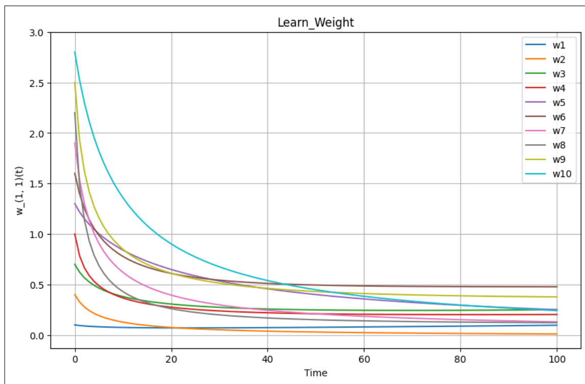
図 2.4: 数値実験
