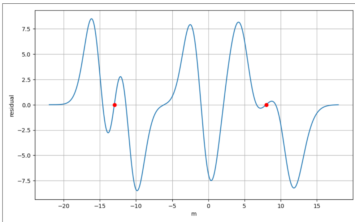
図 2.2: 数値実験
