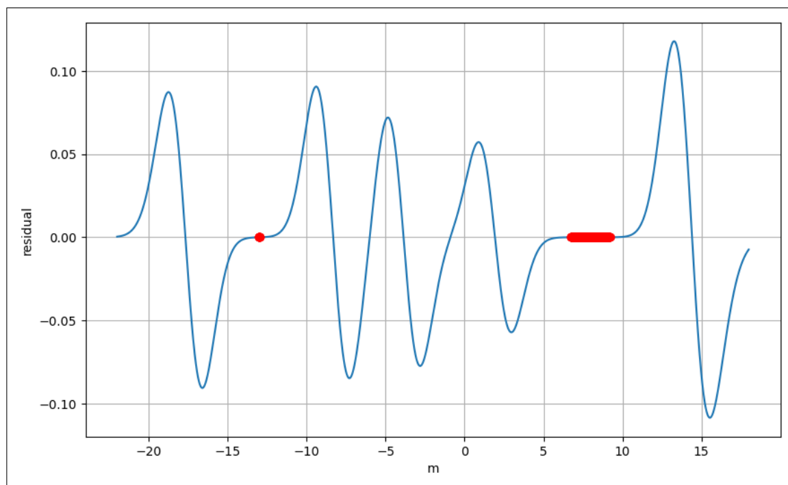
図 2.3: 数値実験
