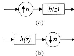
図 1 データの拡大と縮小．拡大 (a) はアップサンプラーとフィルタリングの連続，縮小 (b) はフィルタリングとダウンサンプラーの組合せとみなされる
