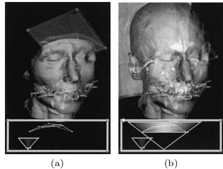
図 11 輝度とこう配の大きさの 2 次元ヒストグラムを使った伝達関数エディタとテクスチャペーストボリュームレンダリング. (from [106], © 2001 IEEE)
