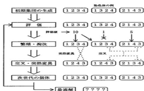
図 4.1: 遺伝的アルゴリズムのイメージ [24]
