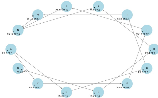
図 3.3: PERT 図 [34]
