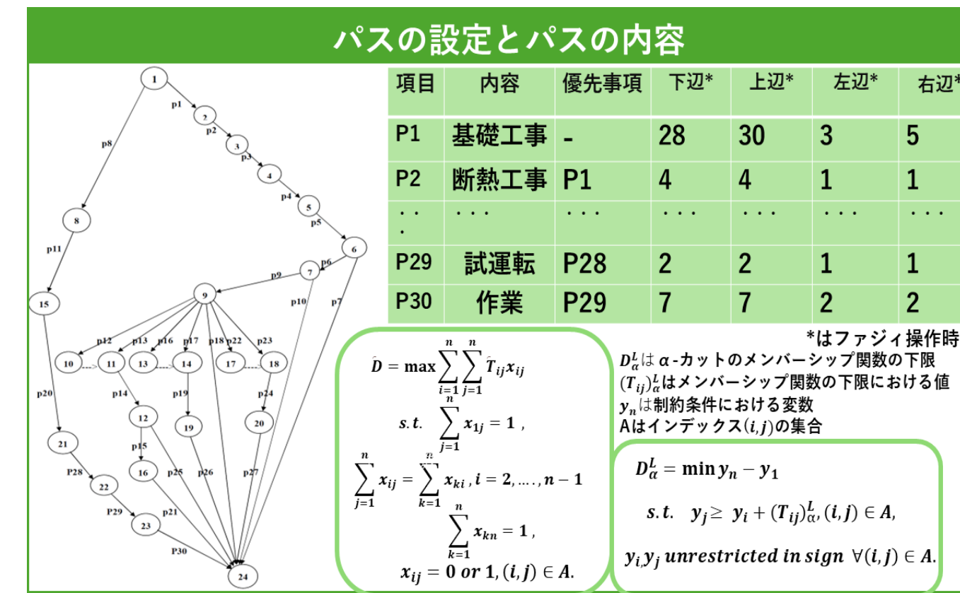
図5 パスの設定
