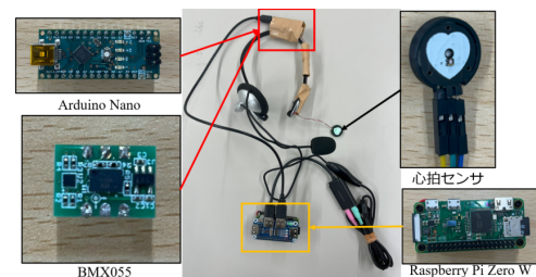
図 3.8: 本研究のネックバンド型機器
