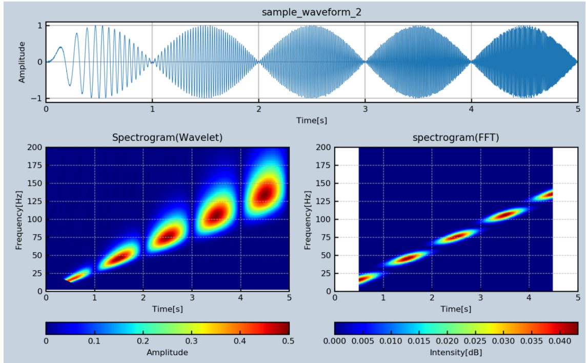
図 2.1: CWT によるスペクトログラム [?]
