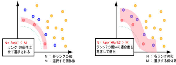
図 3.1: 混雑度トーナメント選択のイメージ
