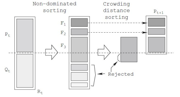
図 3.2: NSGA-II の流れ
