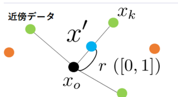
図 4.2: SMOTE のイメージ
