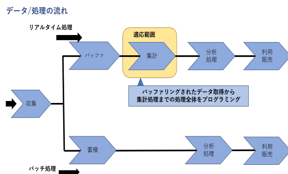
図 4.2: バッチ処理とリアルタイム処理
