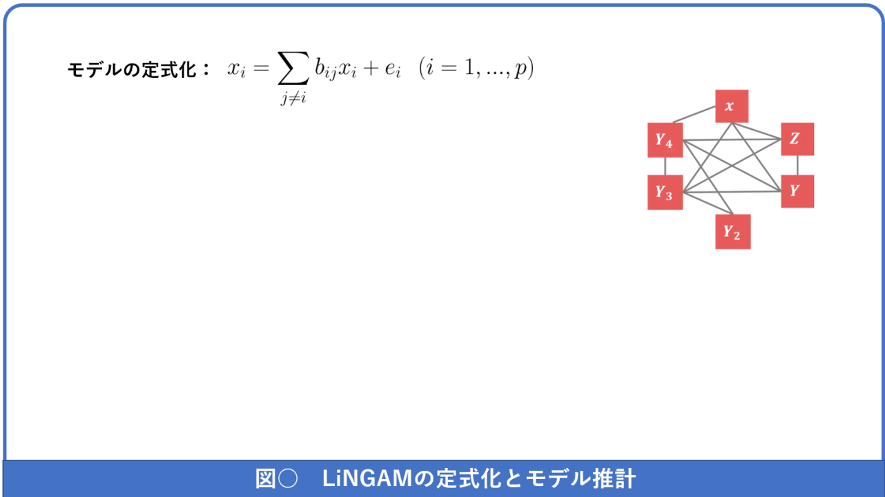
図4 LiNGAMの定式化とモデル推計
