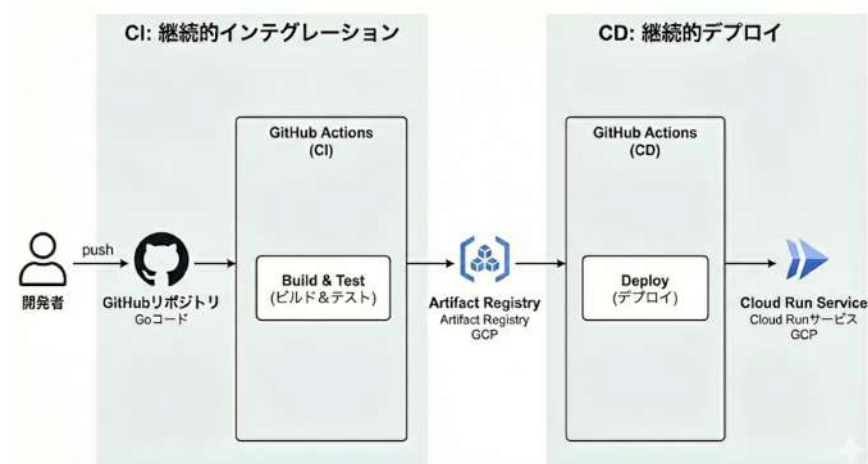
図 2.7: GitHub Actions による CI/CD パイプライン
