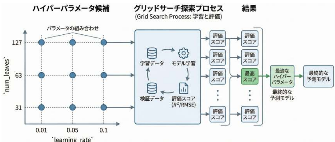
図 3.5: ハイパーパラメータ最適化の概念
