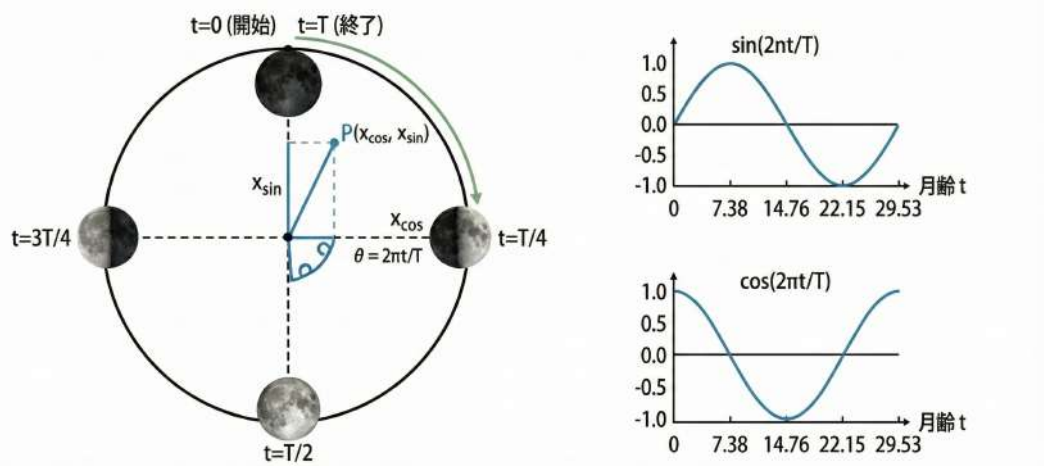
図 3.3: 三角関数を用いた周期的データの表現
