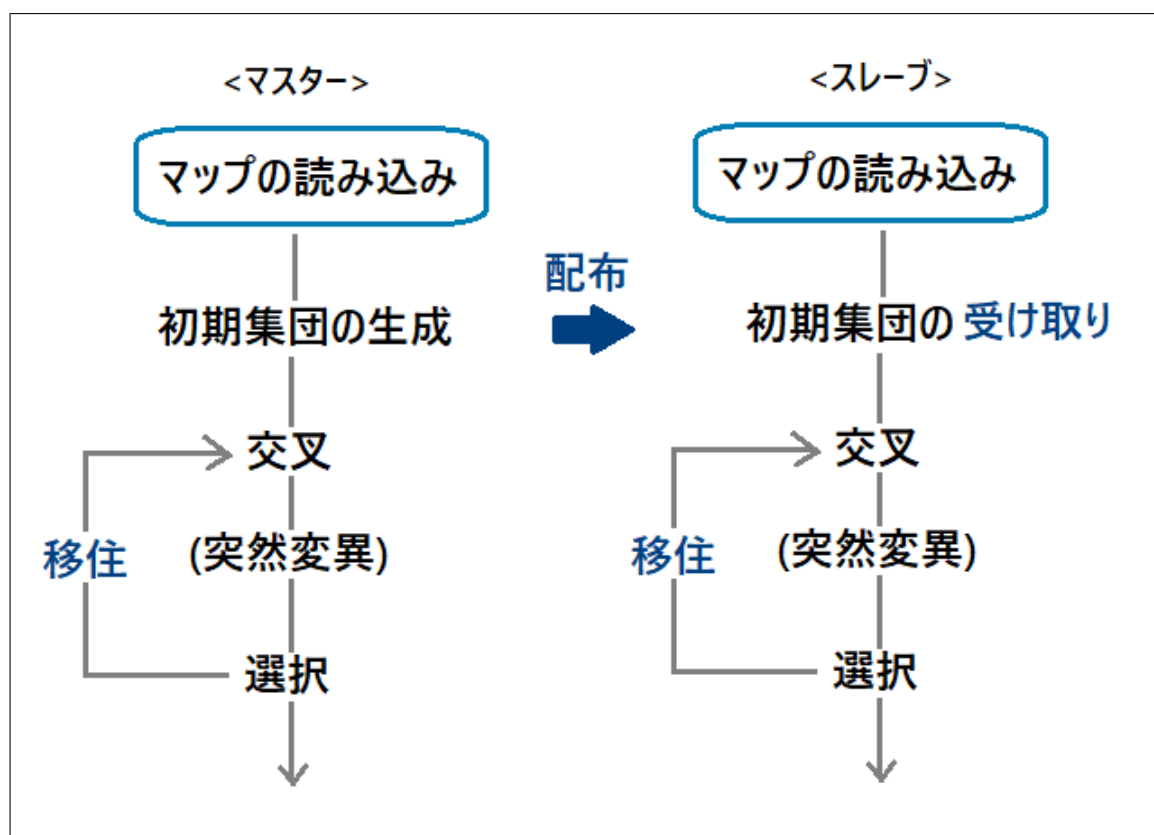
図 3.11: MPI による並列分散 GA のフロー
