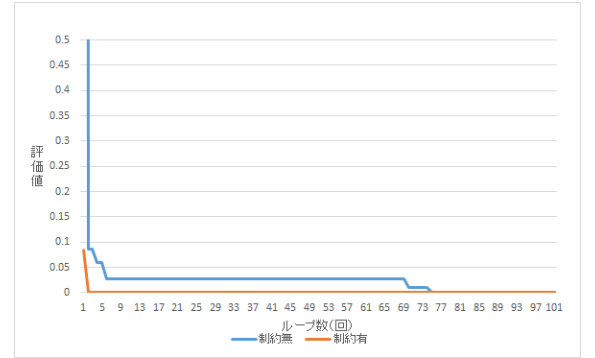
図 4 Rastrigin function の実験結果
