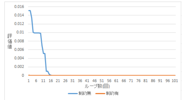
図 5 Griewank function の実験結果
