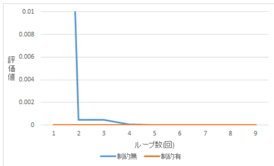
図 7 Matyas function の実験結果
