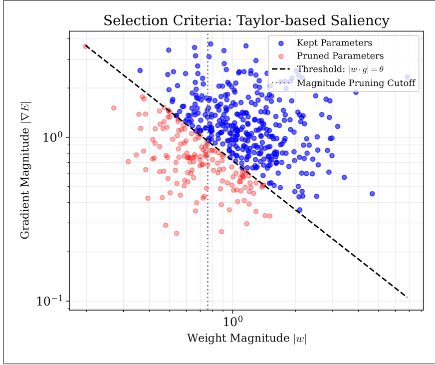
図 4.2: サリエンシーに基づく選別基準
