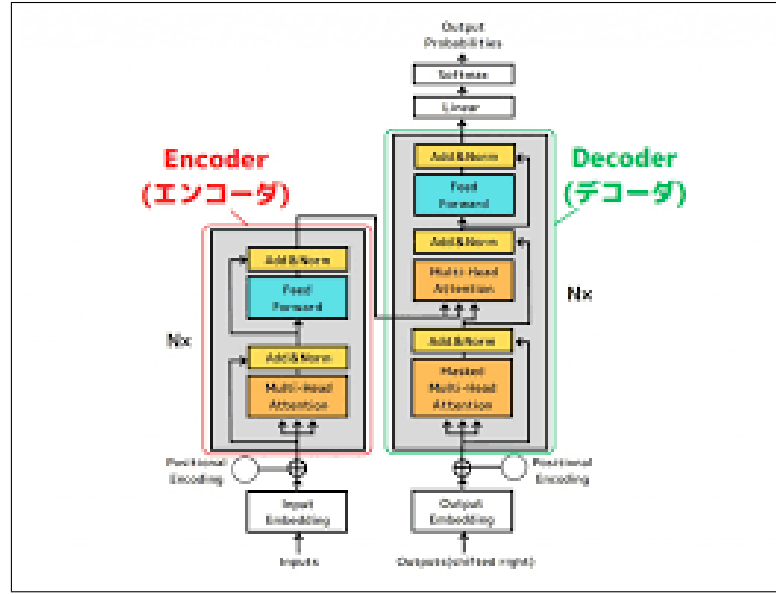
図 3.1: Transformer
