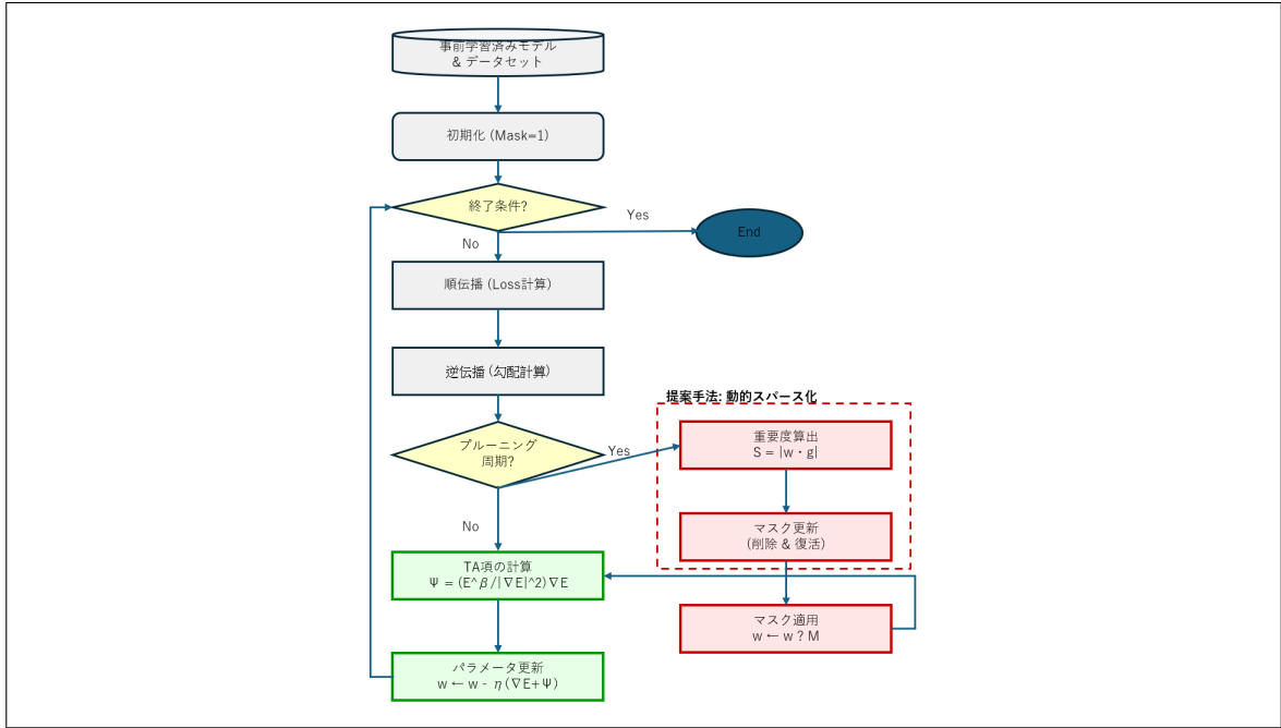
図 4.1: アルゴリズムフロー図
