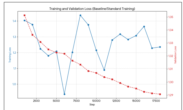
図 5.2: ベースライン損失
