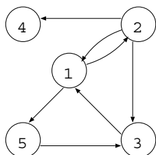
図1 うわさの伝播モデルの有向グラフによる表現．頂点の数字は頂点の番号を表す
