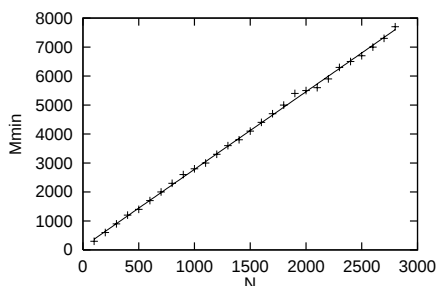
図 4 頂点数 N と非拡散相から拡散相へと転移する最小の弧の数 M_{min} の関係．実線は最小 2 乗法で求めた回帰直線 M_{min} = 2.678N + 102.381
