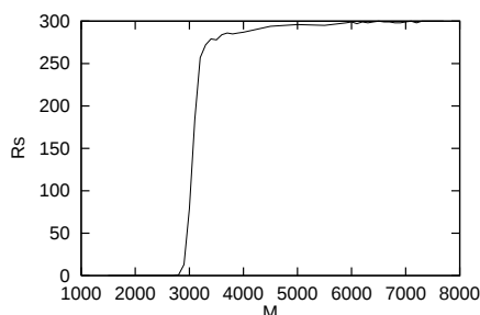
図 2 弧の数 M と蔓延状態になった試行回数 R_s の関係．全試行回数は 300，頂点数 N = 1200 ， \Delta M = 100
