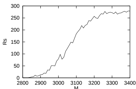
図 3 弧の数 M と蔓延状態になった試行回数 R_s の関係．全試行回数は 300，頂点数 N = 1200 ， \Delta M = 10
